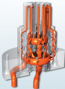
Przekrój wkładki z chłodzeniem konformalnym
